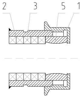
Abbildung 3: Typ SGK
