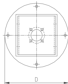
Abbildung 1: Isolier-Rosette
