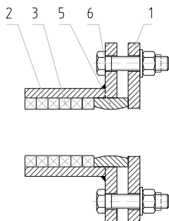
Abbildung 5: Typ SGB
