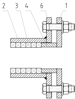
Abbildung 4: Typ SDB
